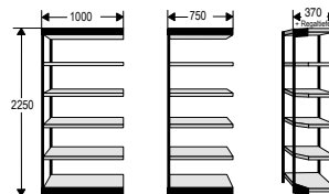
2250 mm hoch und 6 Fachböden
