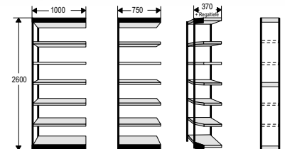
2600 mm hoch und 7 Fachböden
